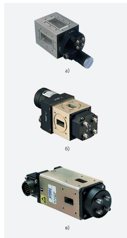
Рис.32. Коаксиально-волноводные DPDT-переключатели компаний Logus Microwave (а, б) и SIVERS (в)
