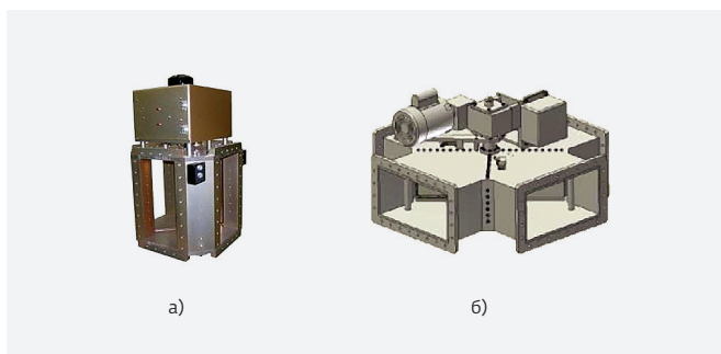
Рис.30. Мощные волноводные переключатели для передатчиков: а – радиовещательных (компания ERI), б – телевизионных (компания Micro Communications)
